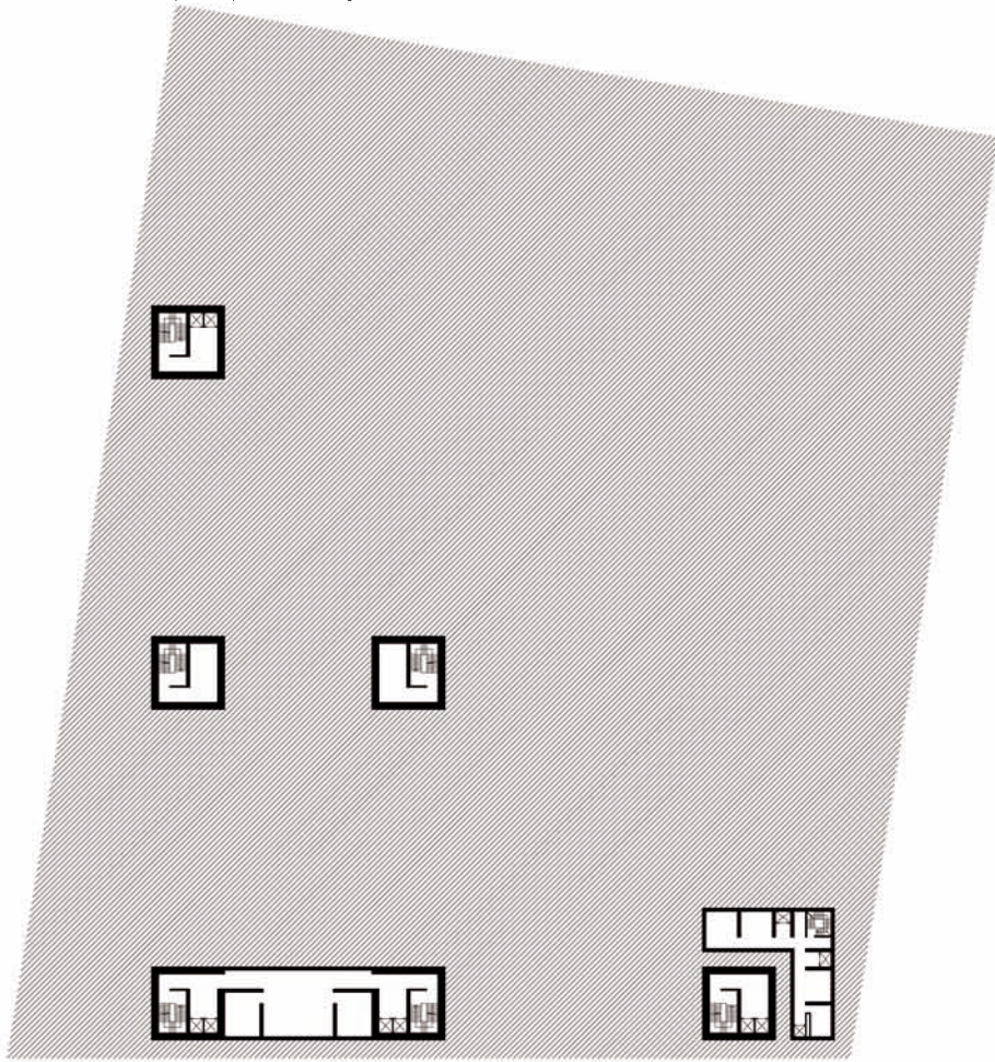
pianta alla quota -4.00 mt in scala grafica 1:500
