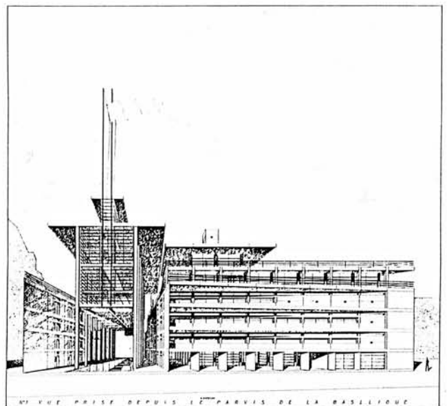
Progetto per l'ampliamento dell'Hôtel de Ville a Saint Denis (Francia), 1985. Coll.: S. Cardon, A.L. Deshaudel, P. D'Incecco, D. Fevre, G.L. Gau- cher, E. Pozzo
