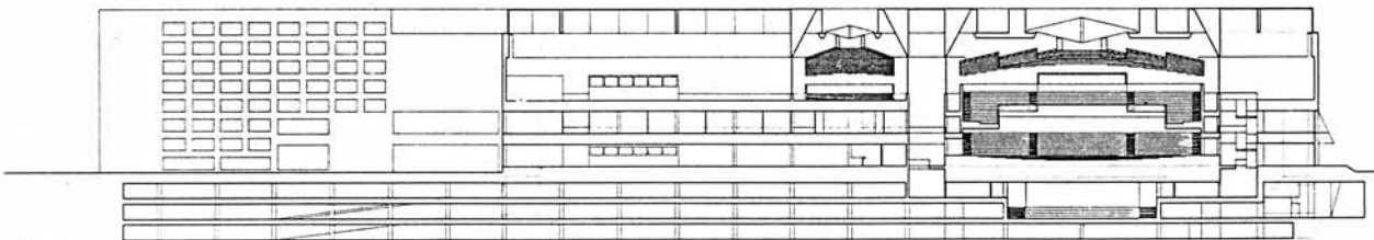
Sección Longitudinal / Longitudinal section
