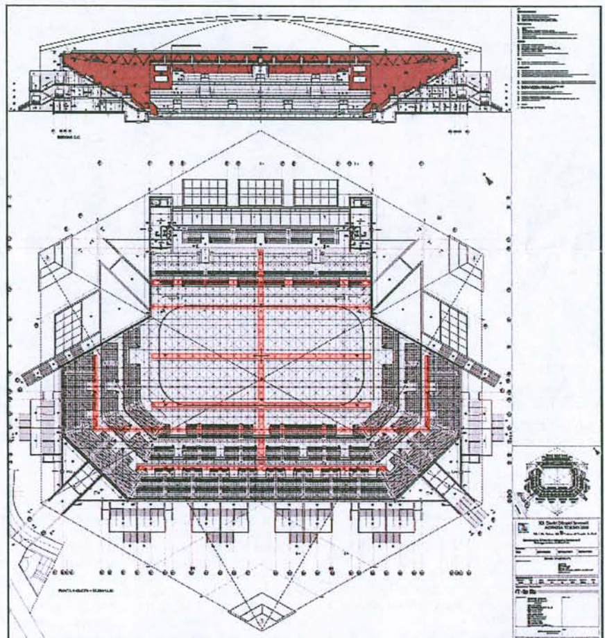
Gae Aulenti, Palavela, Torino - Pianta quota +11,80 e Sezione C:C scala 1: 200, stampa su carta, 2006
